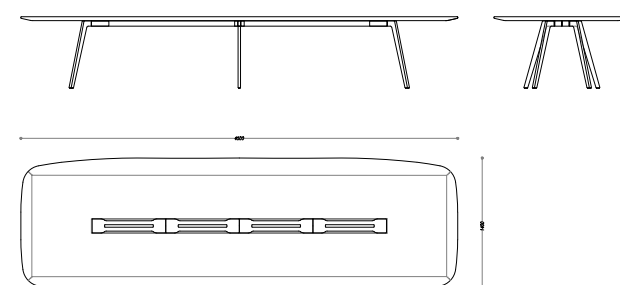
WI450 450x140 cm table - tavolo 450x140 cm
