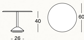
BA20 Tavolino Altezza 60 cm Side-table Height 60 cm Table d'appoint Hauteur 60 cm Beistell-Tisch Hoehe 60 cm
