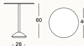
BA10 Tavolino Altezza 40 cm Side-table Height 40 cm Table d'appoint Hauteur 40 cm Beistell-Tisch Hoehe 40 cm
