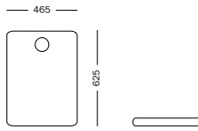
MODULO T1 - Tavolo piccolo rettangolare, 2 prese USB, ricarica wireless MODULE T1 - Small rectangular table, 2 USB plugs, wireless recharge system
