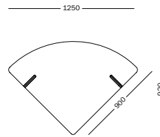
MODULO F - Modulo angolare 90° MODULE F - 90° angular module
