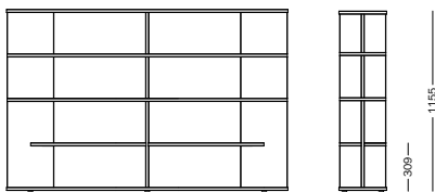
MODULO 4 - Libreria alta MODULE 4 - High bookshelf
