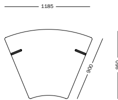
MODULO C - Modulo angolare 45° MODULE C - 45° angular module
