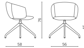
NT 4096 MINI mini-armchair, swivel polypropylene base poltroncina mini, base girevole in polipropilene
