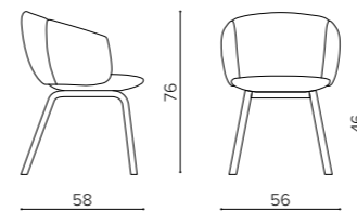
NT 4094 MINI mini armchair, wooden base poltroncina mini su base a 4 gambe in legno
