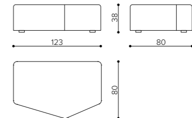
ST D00L left module D modulo D sinistro module D gauche
