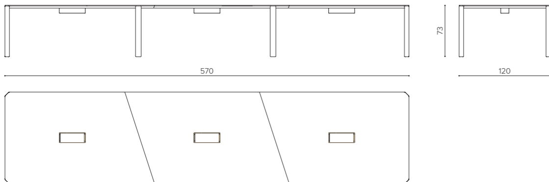
ER 570120 table 570x120cm tavolo 570x120cm table 570x120cm
