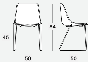
Sled base
