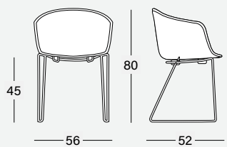
Sled base
