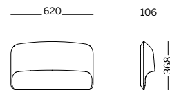
MODULE 5 - Right high armrest MODULE 6 - Left high armrest
