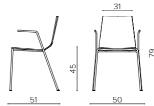
MA 104T 4 legs steel rod base chair with armrests sedia a 4 gambe in tondino d'acciaio con braccioli chaise en fil d'acier à 4 pieds avec accoudoirs
