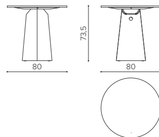
NM 8074 Table Ø80 Tavolo Ø80 Table Ø80
