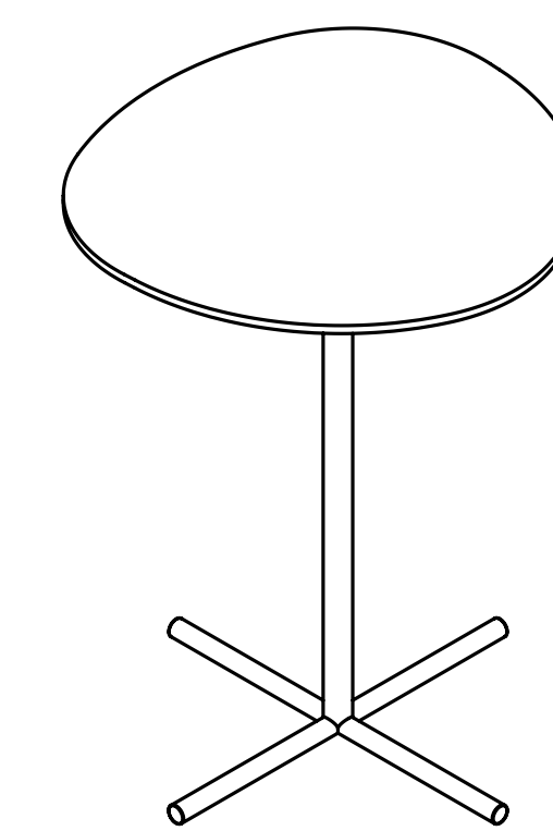
NTT0105T W78,7 · D76,7 · H105
