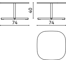
NTT00S low square table h40 cm tavolo quadrato basso h40 cm table basse carrée h40 cm
