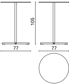
NTT0105R high circular table h105 cm tavolo circolare alto h105 cm table circulaire haute h105 cm
