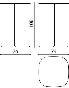
NTT0105S high square table h105 cm tavolo quadrato alto h105 cm table haute carrée h105 cm
