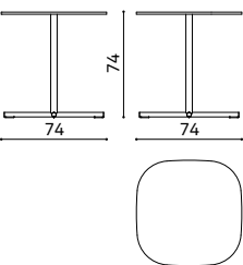
NTT0HS square table h74 cm tavolo quadrato h74 cm table carrée h74 cm
