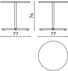
NTT0HR circular table h74 cm tavolo circolare h74 cm table circulaire h74 cm
